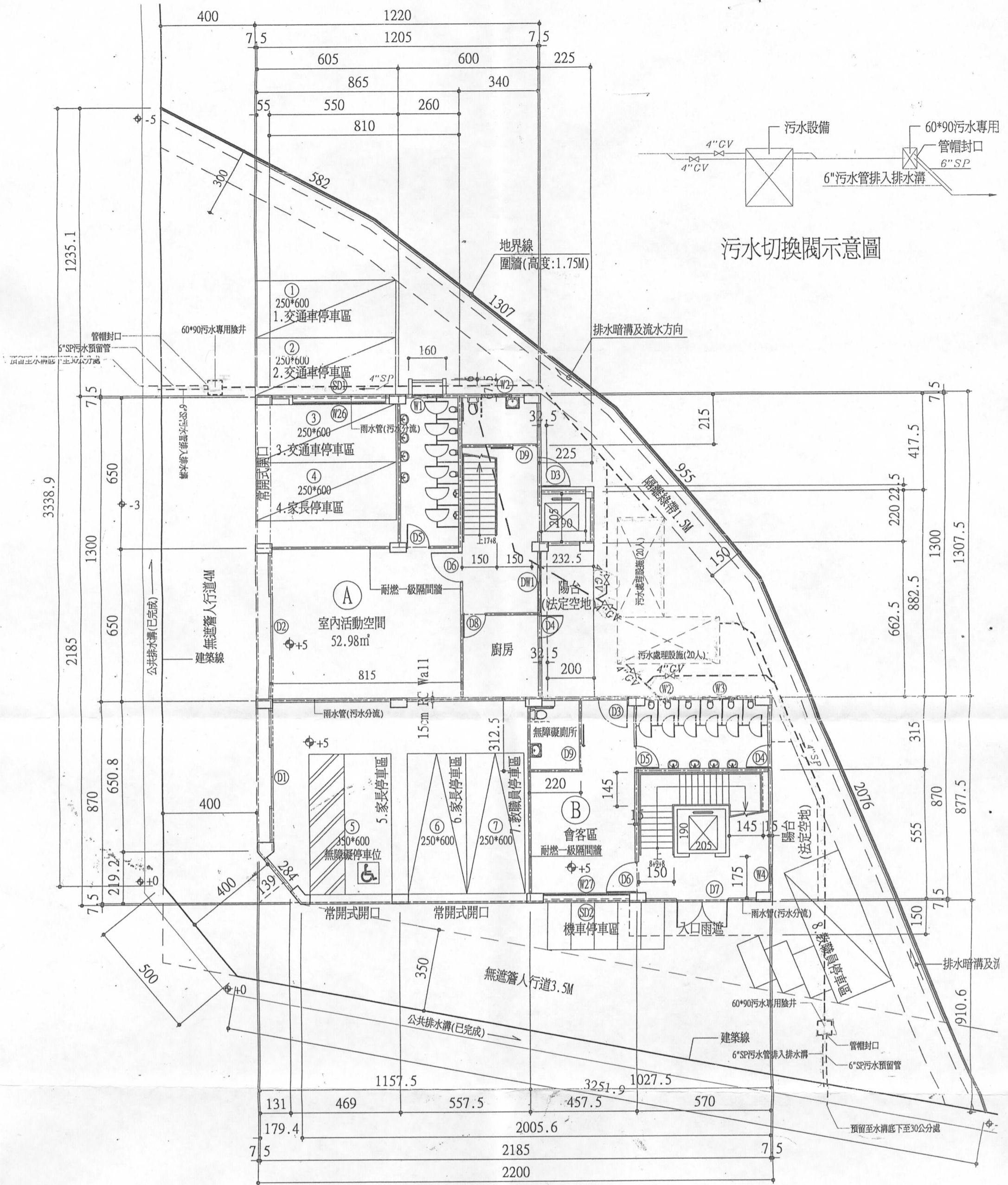
壹層平面圖 S:A1=1/100;A3=1/200
