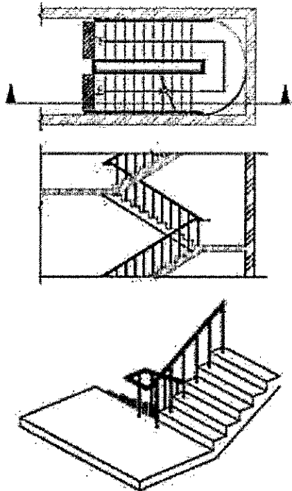
扶手與平台欄杆，其平台寬度，應與梯段寬度一致。
