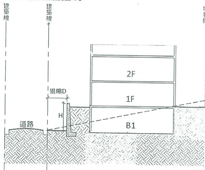
(七)擋土設施量體控制
