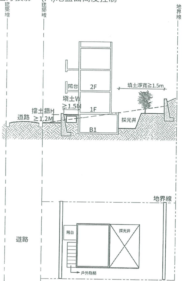
(五)上方投影、(六)地盤面高度控制
