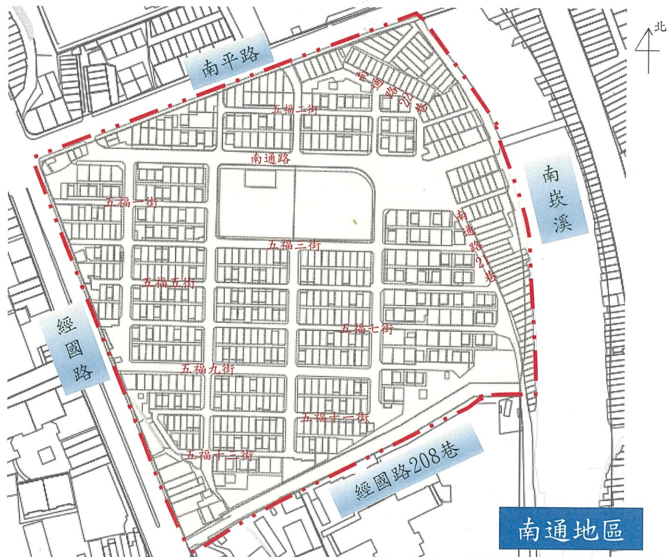
桃園市桃園區污水下水道系統分支管網範圍圖
