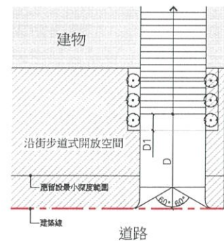
(3) 起降點突出於外牆外緣
