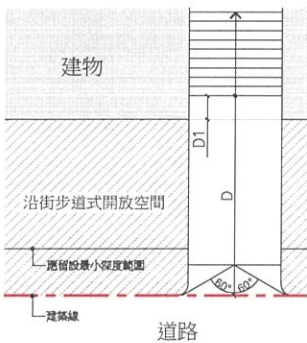
(1) 起降點位於外牆外緣內
