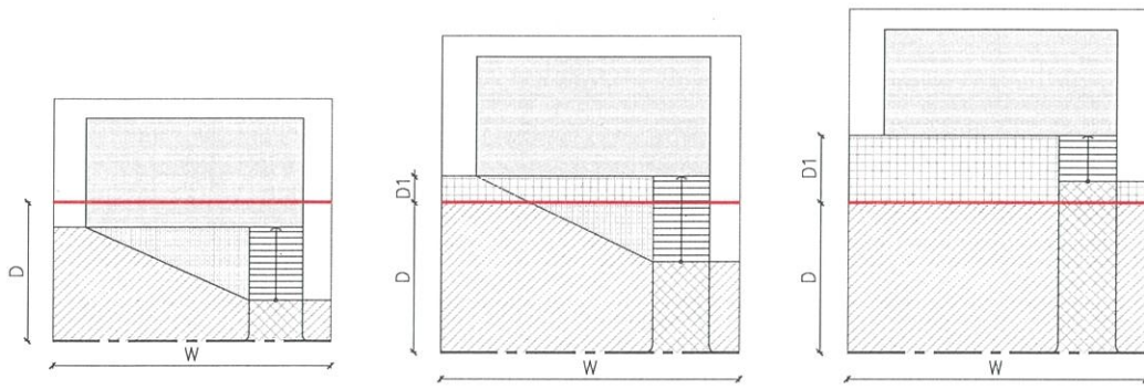
圖十之二 有效係數計算
