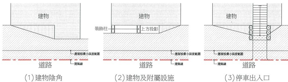
圖十之一 開放空間連線及係數檢討
