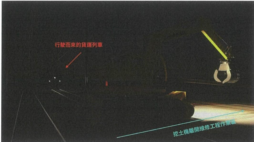
圖 7. 貨運列車撞擊正在離開作業區的挖土機
