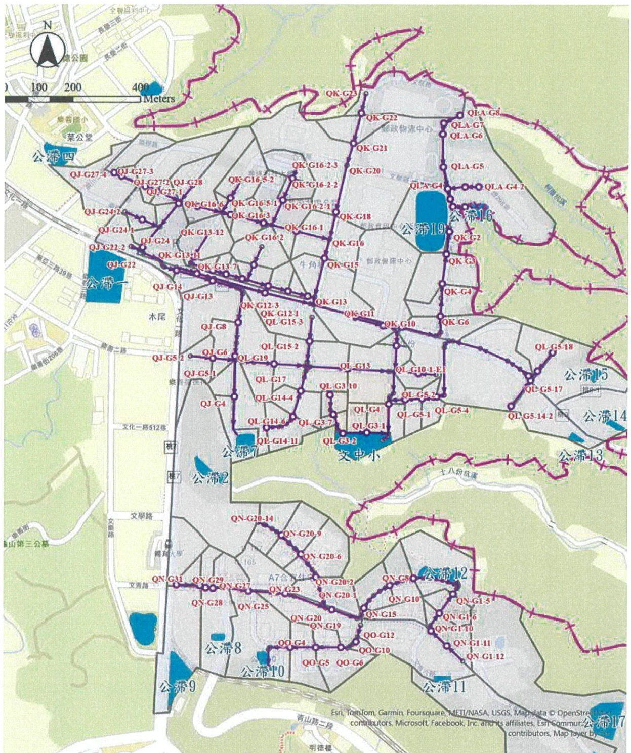
公告雨水下水道幹(支)線編號圖
