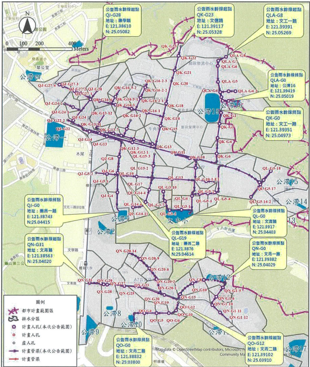
公告雨水下水道排水區域範圍圖
