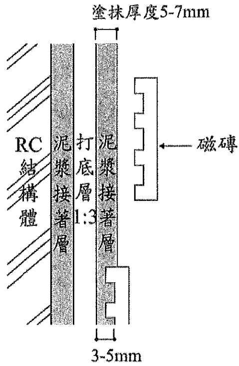
圖 9 壓貼工法
