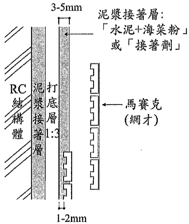
圖 10 才貼工法
